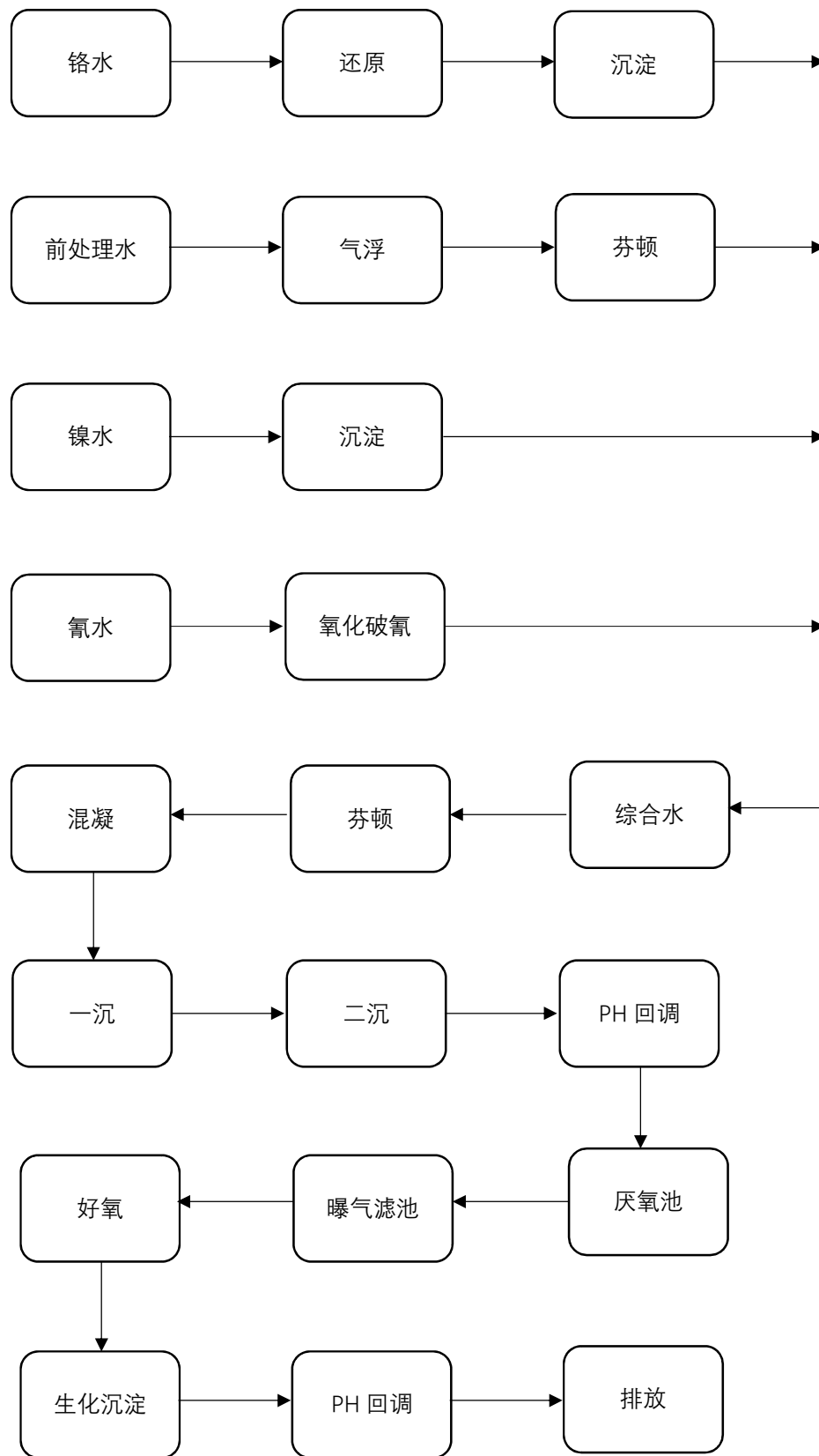
鹰松五金塑胶制品有限公司废水处理流程
